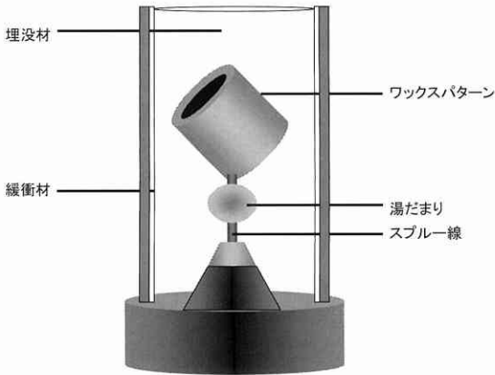
図2 埋没後における鑄造リングの模式図
