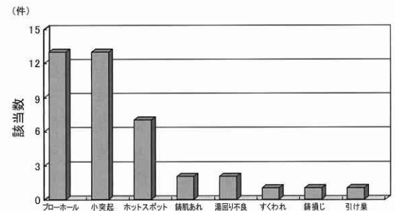
図6 鑄造欠陥の観察
