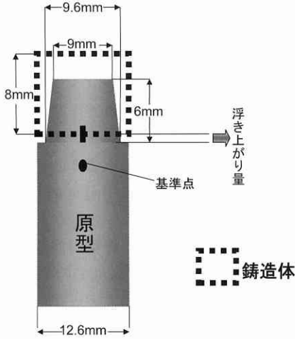
図1 支台原型および鑄造体
