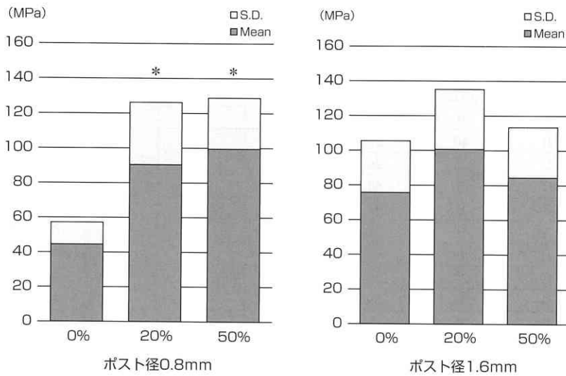
図6 AFFのフィラー配合率と抗折強さ(メラミン歯, シリンダー型)
