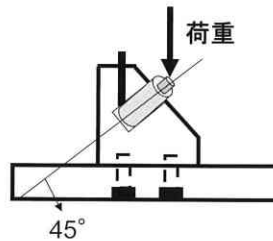
図2 抗折強さの測定
