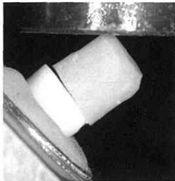
図3 抗折試験の状況
