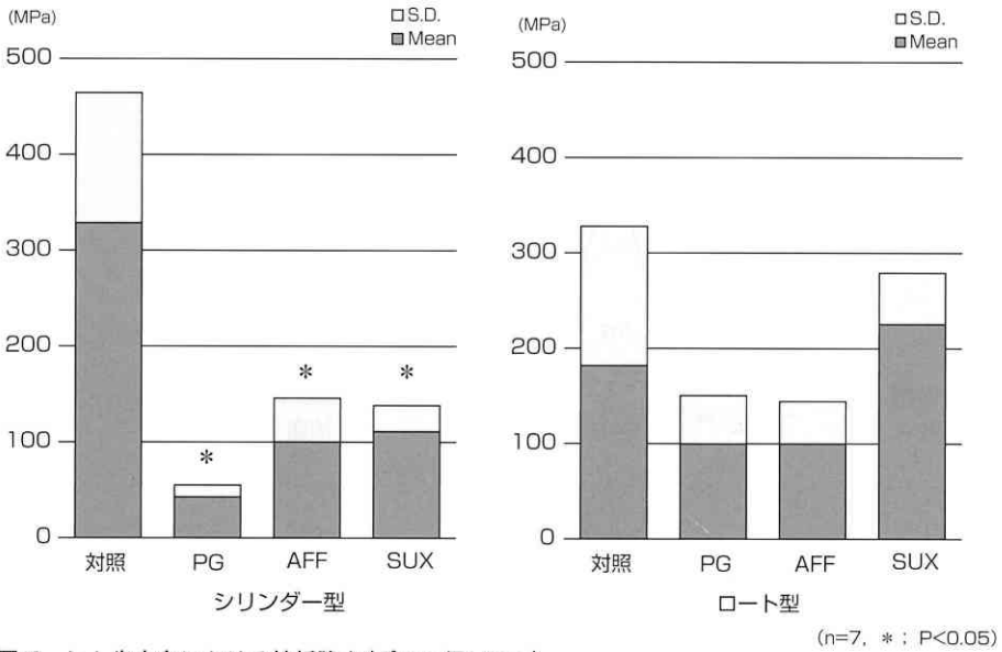
図10 ヒト歯支台における抗折強さ(ポスト径1.6mm)
