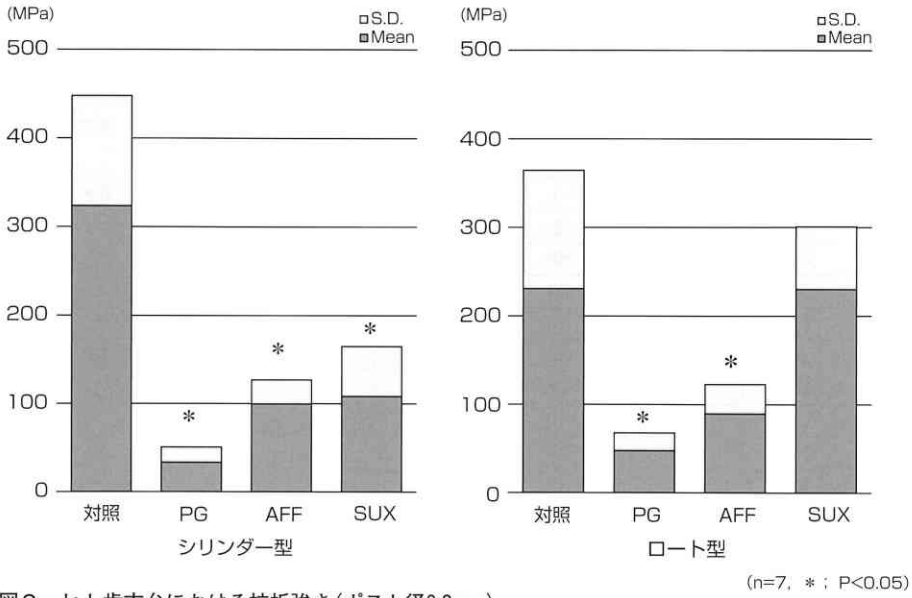
図9 ヒト歯支台における抗折強さ(ポスト径0.8mm)
